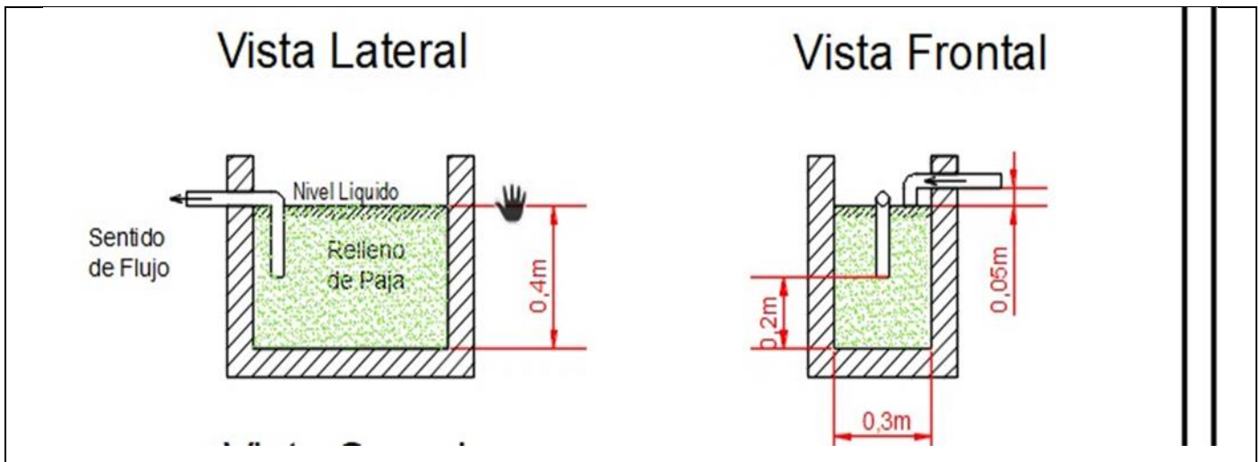
Imagen 11 - Detalle clarificador de paja
