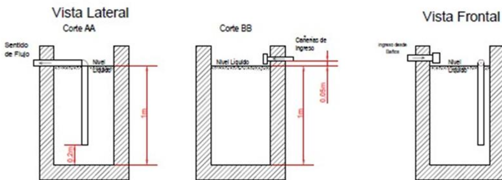
Imagen 8- Detalle grasera
