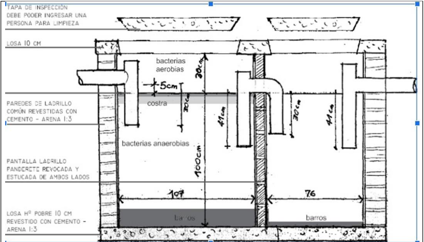
Imagen 2 - Cámara Séptica – Corte Transversal - Detalles constructivos
