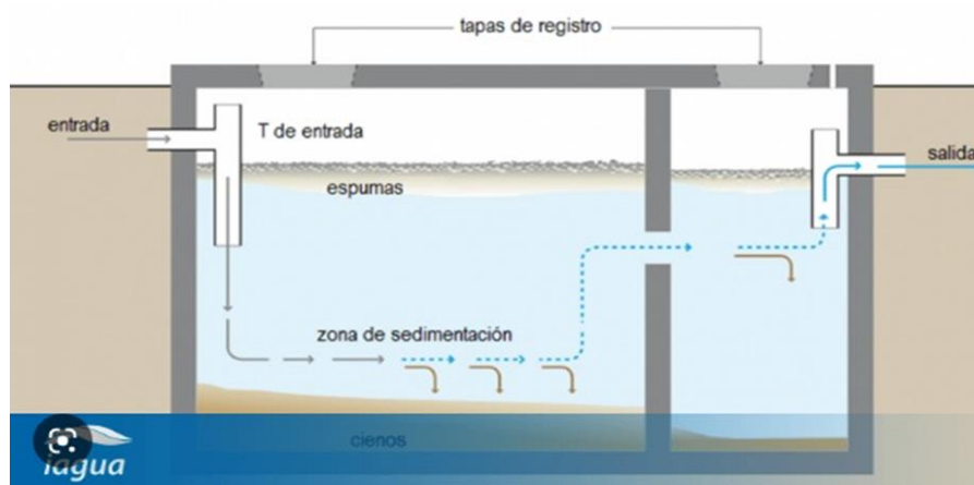
Imagen 1 - Ejemplo de Cámara Séptica con divisiones internas
